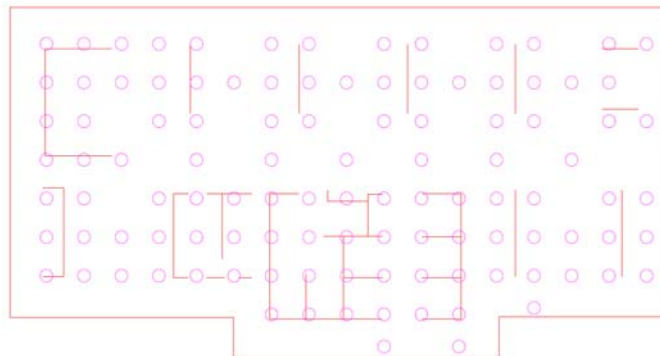
Fig. 12. Pile layout
